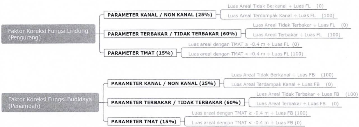
Gambar 2. Diagram Persentase Bobot Untuk Tiap Parameter Penyusun Faktor Koreksi Gambut
